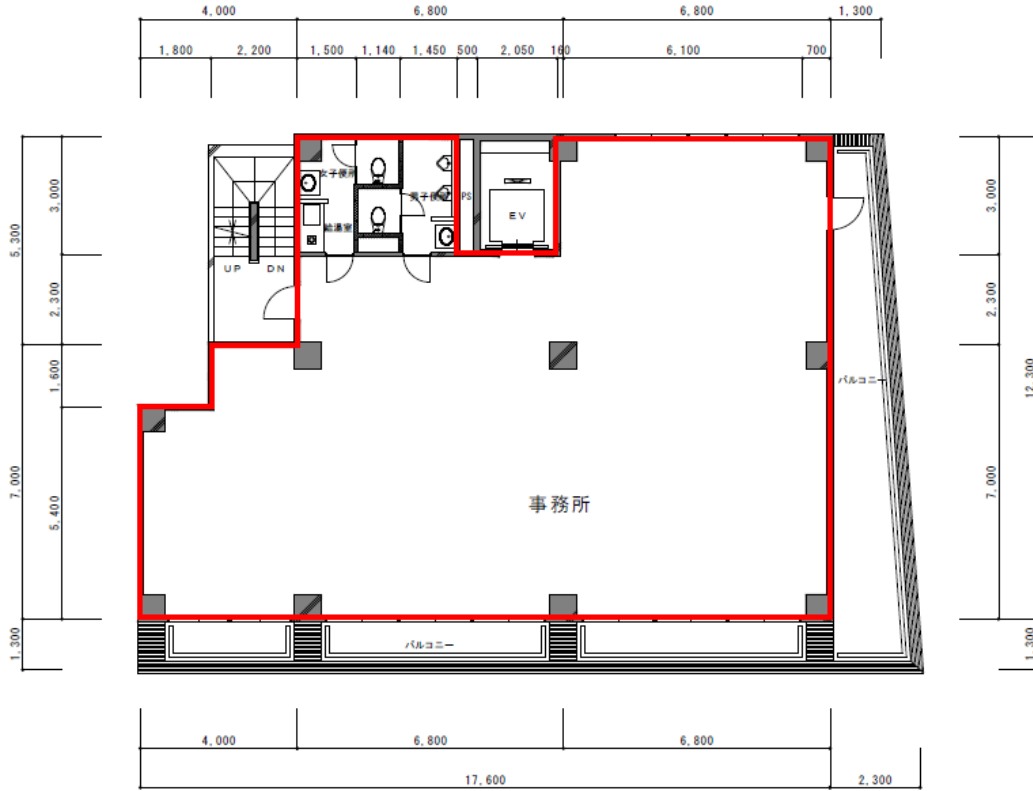
6階平面図
